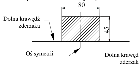
Rys. 2 Wycięcie zderzaka Ford Maverick
